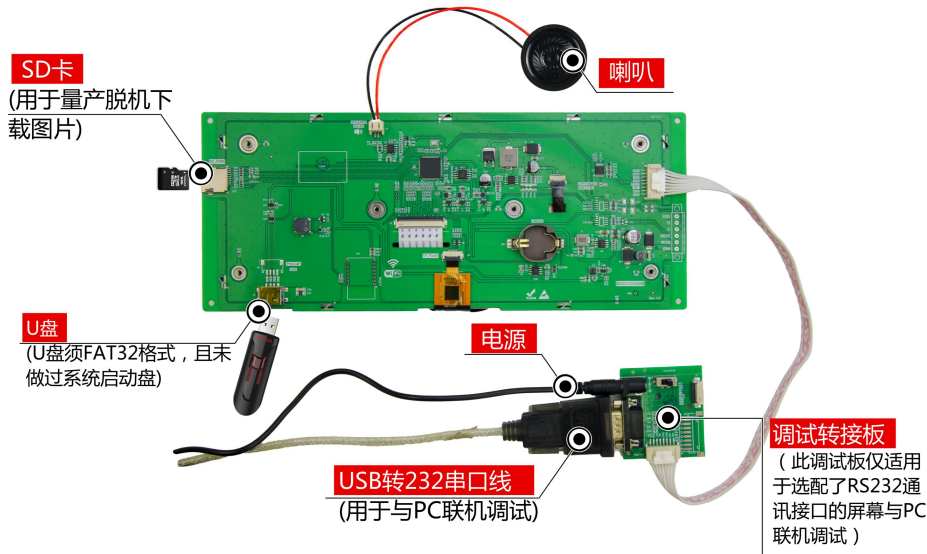
图 1-3 调试工具图
