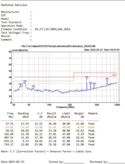
图 5-7 辐射测试垂直方向
