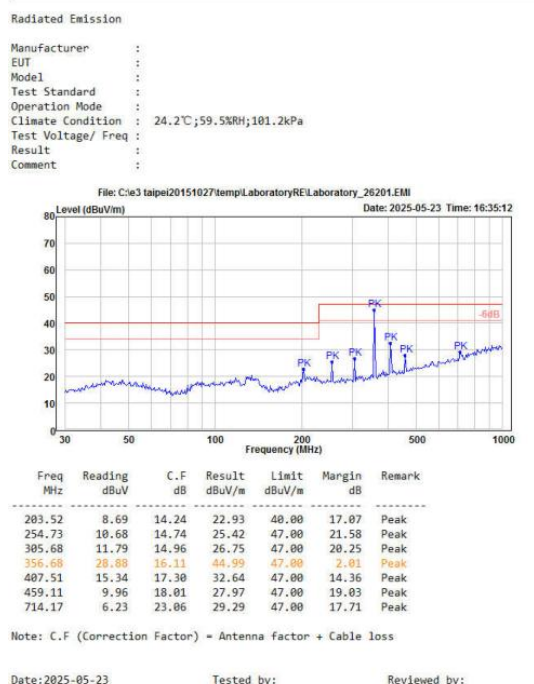
图 5-6 辐射测试水平方向
